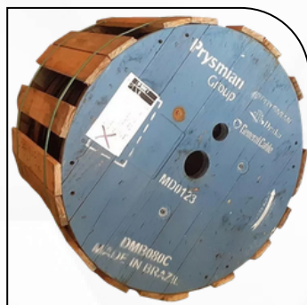
CABO OPTICO DDR-G EXT | 02 À 144FO SM | MM (62,5/125, 50/125 OM2, OM3 E OM4)
